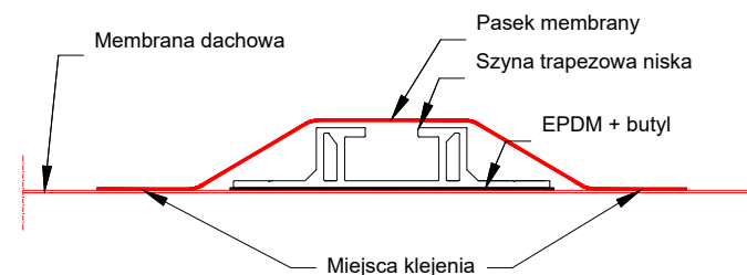
Sposób montażu osłony tylnej
