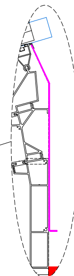
Sposób montażu osłony tylnej
