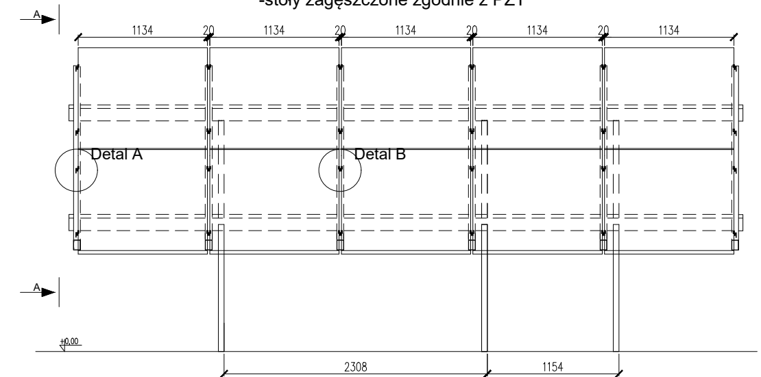
WIDOK W1 - stoły 2x5 - skala 1:50 -stoły zagęszczone zgodnie z PZT
