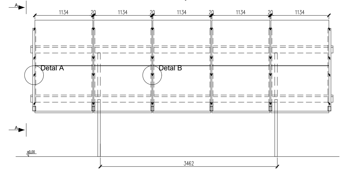
WIDOK W1 - stoły 2x5 - skala 1:50
