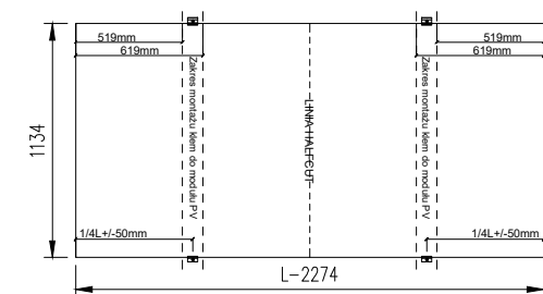
DETAL MONTAŻU KLEM DO MODUŁU FOTOWOLTAICZNEGO Jinko Tiger Pro JKM535M-72HL4-BDVP 525-545Wp Bifacial Halfcut 535Wp o wym. 2274x1134x30mm
