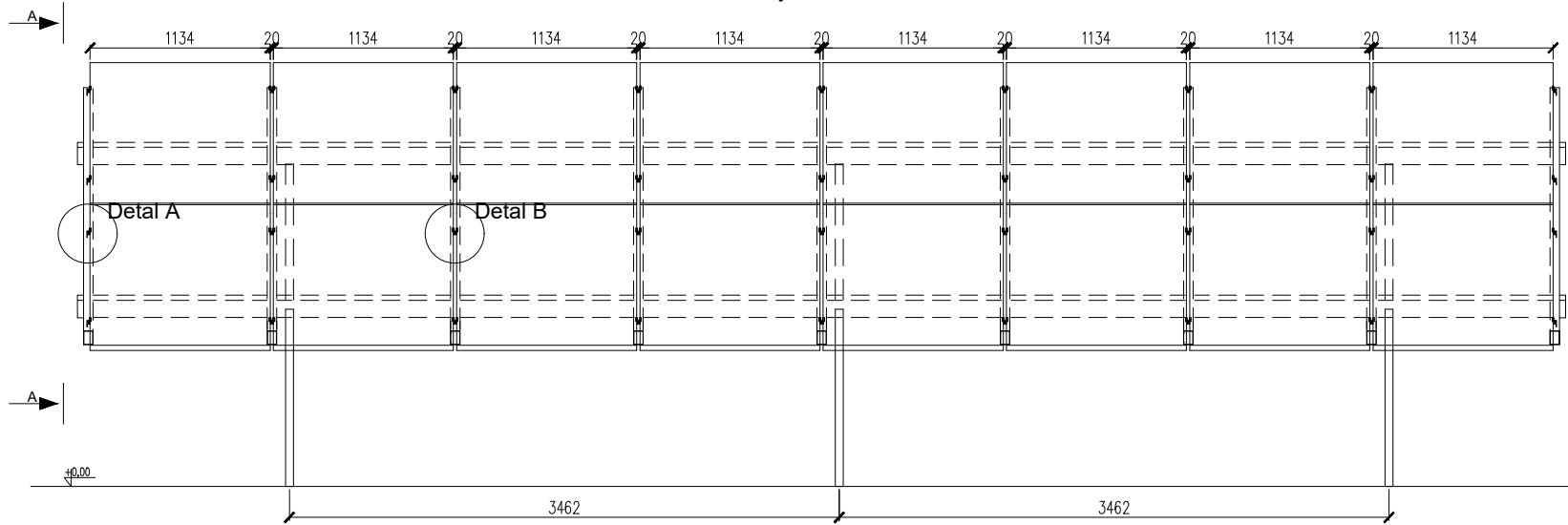
WIDOK W1 - stoły 2x8 - skala 1:50
