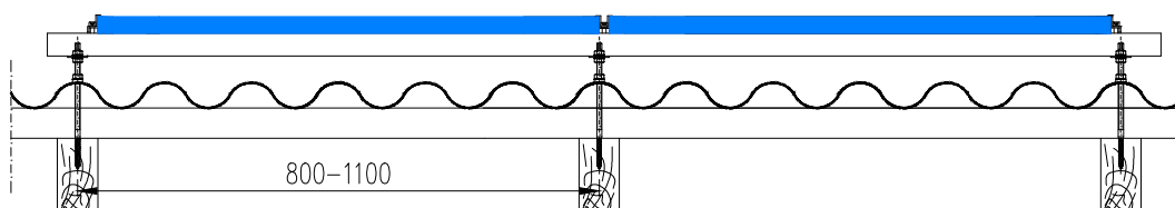
PRZEKRÓJ A-A
