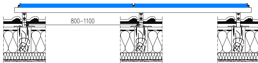
PRZEKRÓJ B-B
