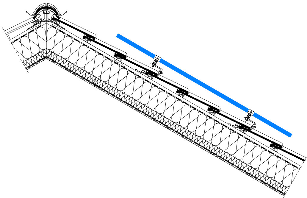
PRZEKRÓJ B-B
