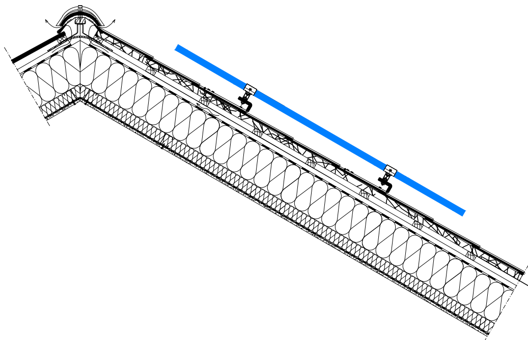
PRZEKRÓJ B-B
