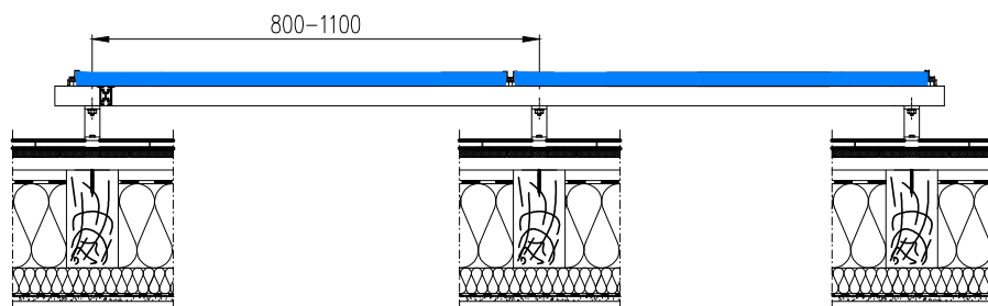
PRZEKRÓJ B-B
